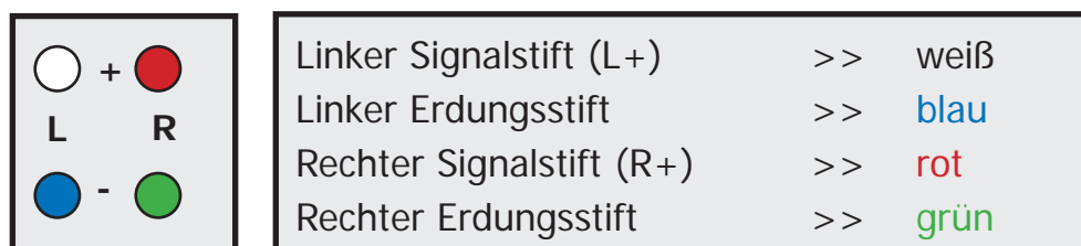
Abb. 1: Farben der Tonarmverkabelung
